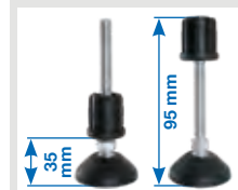
Höhenverstellbare Fußplatte als Sicherheitszubehör erhältlich
