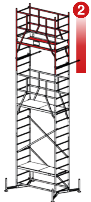
2. Aufstockung Art.-No. 710147 1. Aufstockung Grundgerüst Art.-No. 710123 Art.-No. 710116
