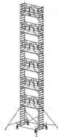
Arbeitshöhe: 14,50 m Standhöhe: 12,50 m Gerüsthöhe: 13,60 m
