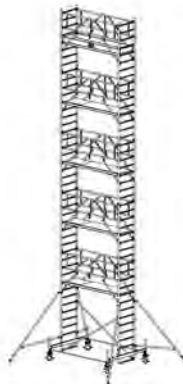
Arbeitshöhe: 12,50 m Standhöhe: 10,50 m Gerüsthöhe: 11,60 m
